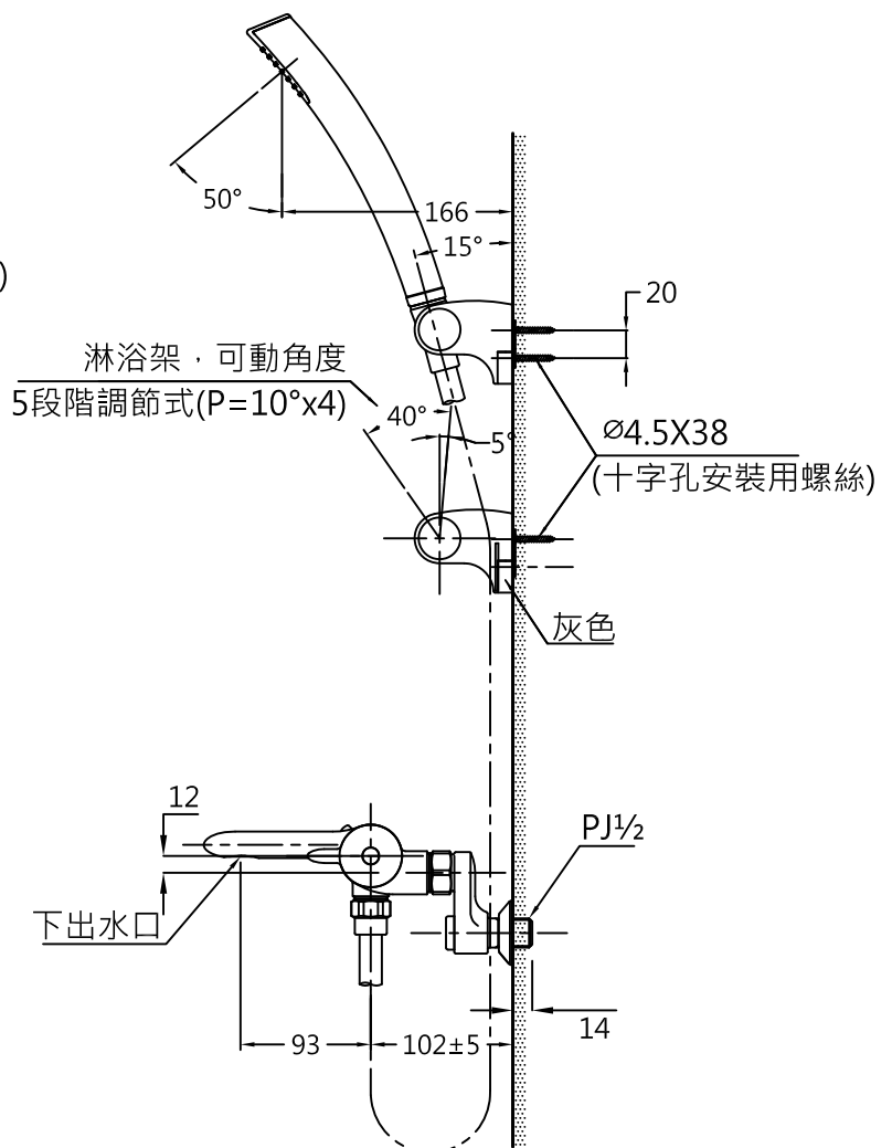
詳細注意標(1:1)
