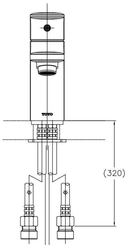
P視圖
