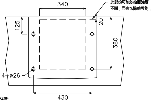
枱面裁切尺寸
