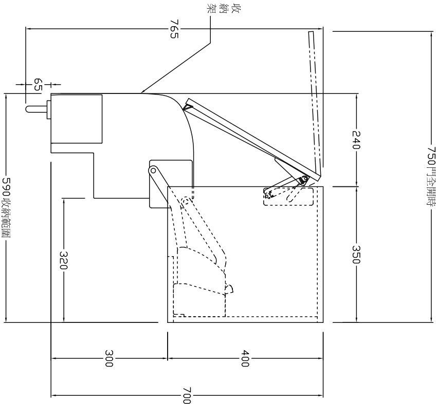
升降浴櫃門詳細尺寸(側面圖)
