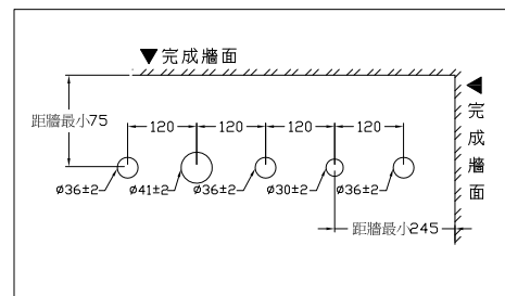
安裝孔徑及尺寸
