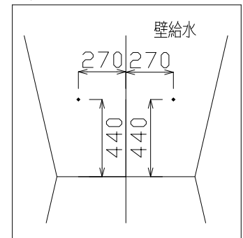
水箱給水取出位置
