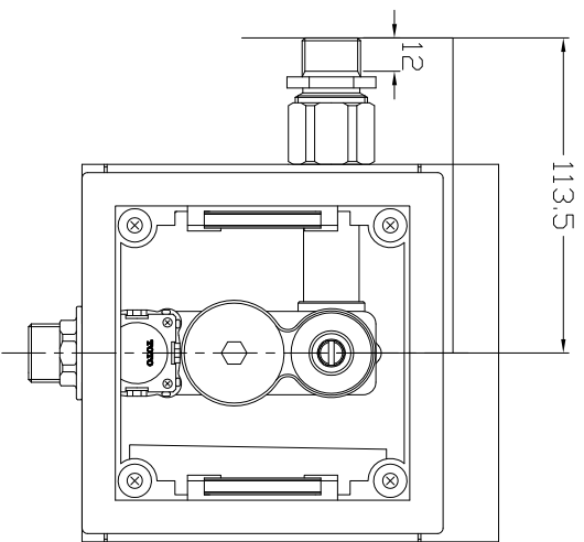
正面透視圖
