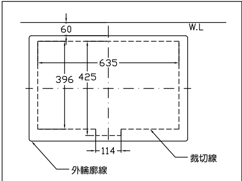
施工板尺寸圖
