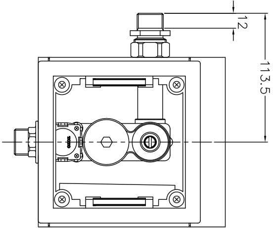
正面透視圖
