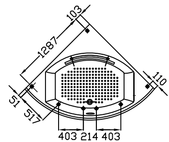
底脚位置图
