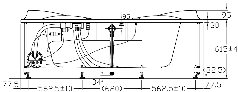
A-A圖面
