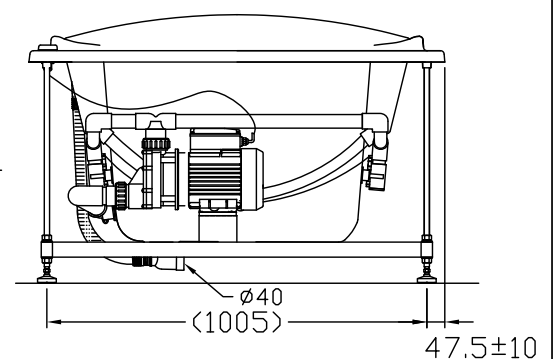
B-B圖面
