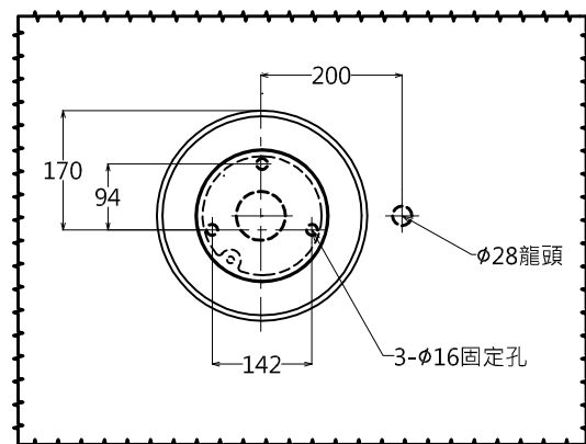
<固定孔徑尺寸圖>
