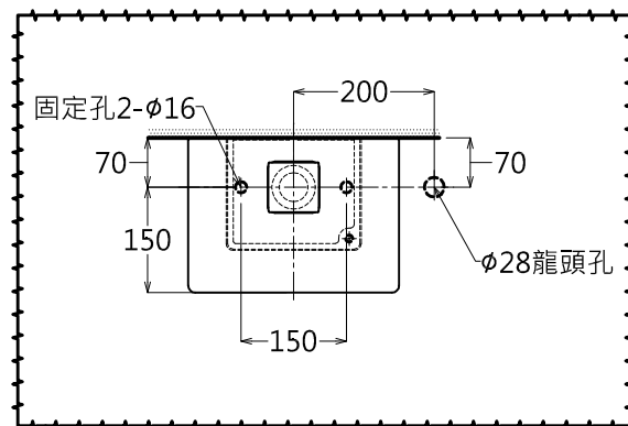
<固定孔徑尺寸圖>
