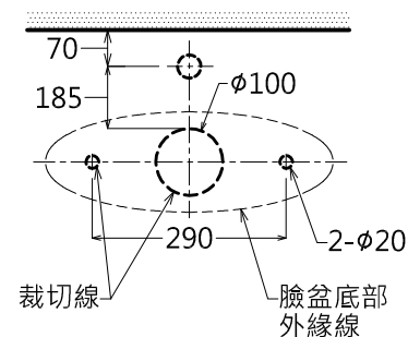
LW818J 檯面裁切尺寸
