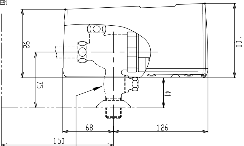
陶瓷水圈面
