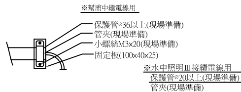
保護管固定部詳細圖
