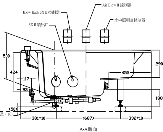
A-A斷面
