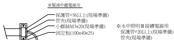
保護管固定部詳細圖
