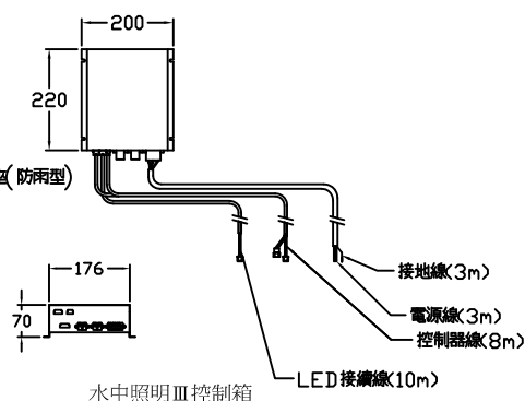
水中照明Ⅲ控制箱
