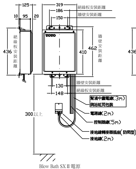
Blow Bath SX II 電源
